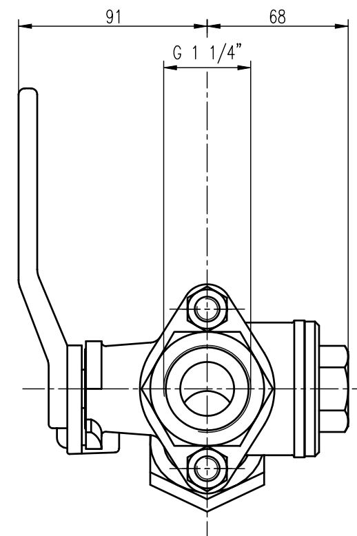
Ansicht A
